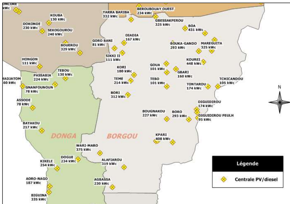
Figure 45: Localisation et puissance des centrales PV - zoom sur DONGA et BORGOU
