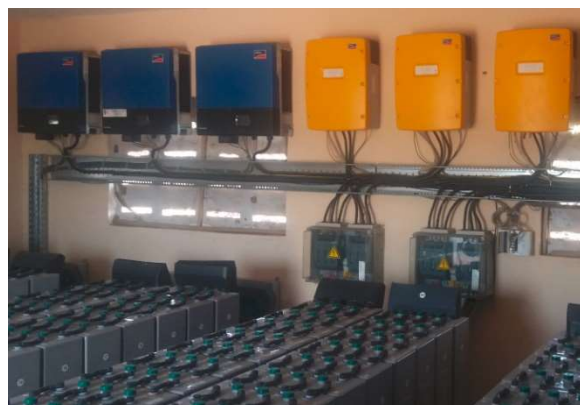
Figure 8: Parc de batteries et onduleurs du système 100% PV de Kabo (Bourgou)
