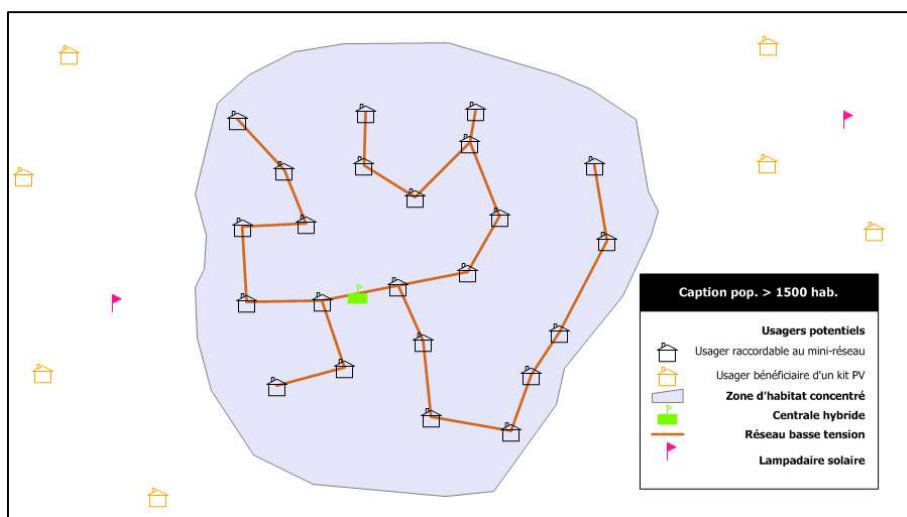
Figure 1: Illustration option technique pour les localités &gt; 1500 hab.
