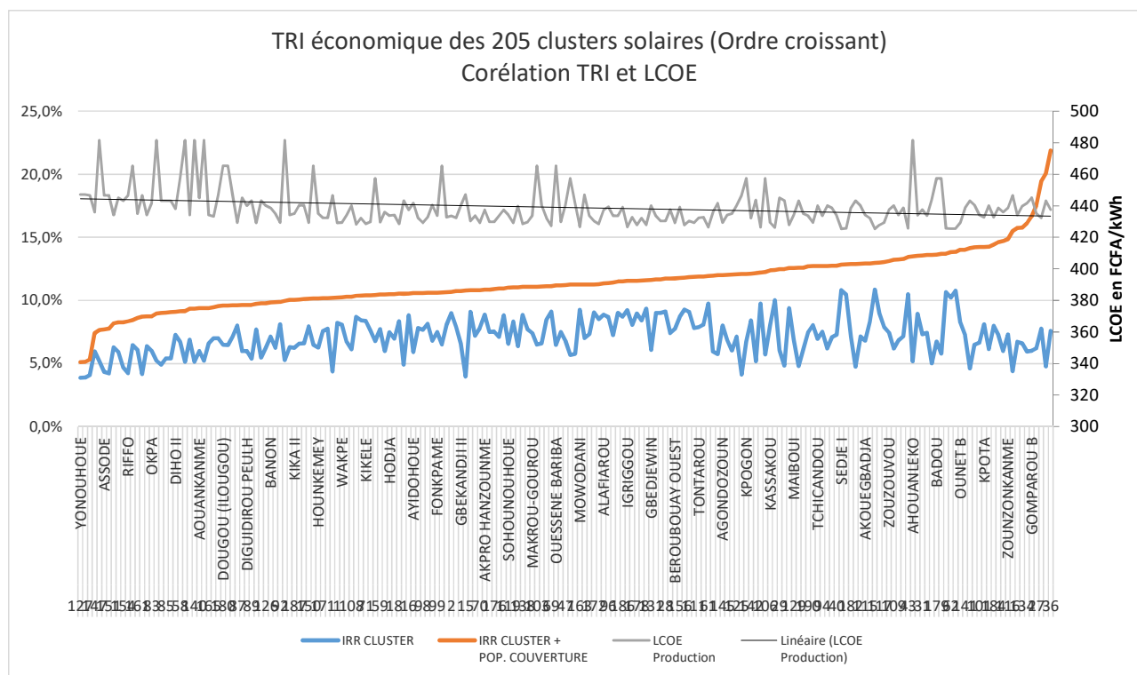
Figure 74 : Taux de rendement économique des 205 projets solaires
