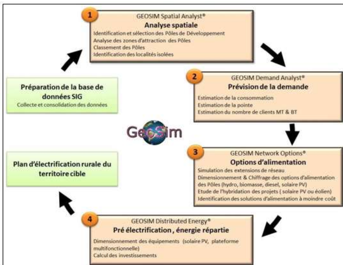
Figure 4: Processus de planification du logiciel GEOSIM®
