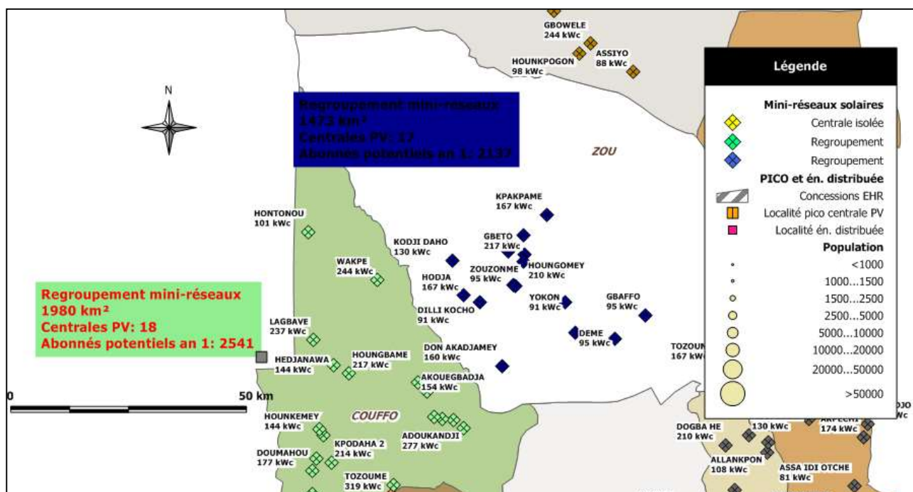
Figure 64: Zoom sur les regroupements potentiels de mini-réseaux – ZOU et COUFFO
