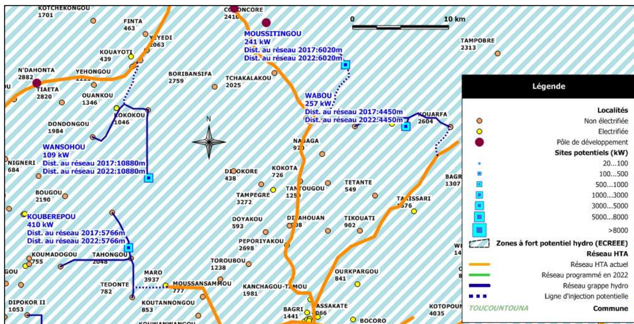
Figure 51: Grappes alimentées par les sites hydro de WANSOHO, MOUSSITINGOU, WABOU, KOUBEREPOU
